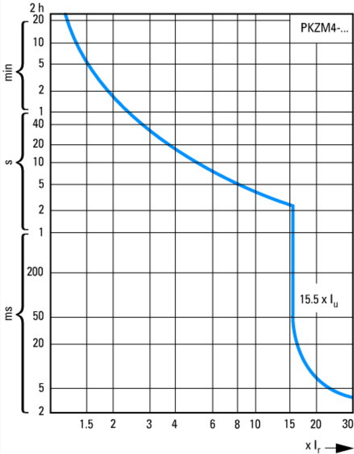
Curve caratteristiche d'intervento
