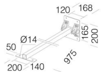
42 braccio orientabile
