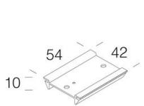
6030 Supporto sezionatore
