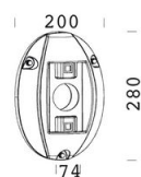
302 Attacco parete
