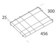
350 Gabbia di protezione - Rodio 36LED
