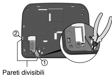
Pareti divisibili
