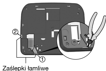
Zaślepki łamielwe
