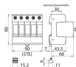
Dimensioni DG M PV2 SCI SN1868
