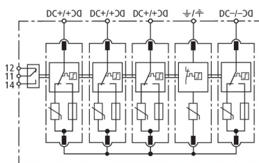
Schema di principio DG M PV2 SCI SN1868
