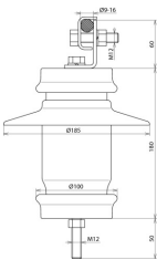
Dimensioni DTR 2.4 10 3
