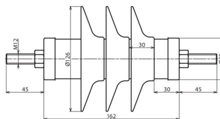
Dimensioni DMI 15 10 1 H
