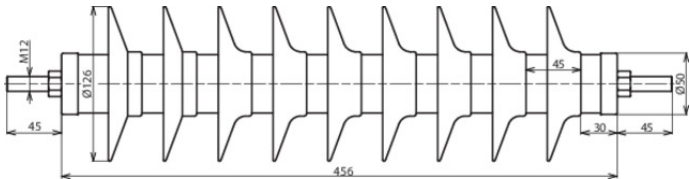
Dimensioni DMI 51 10 1 N
