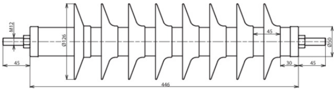
Dimensioni DMI 48 10 1 N
