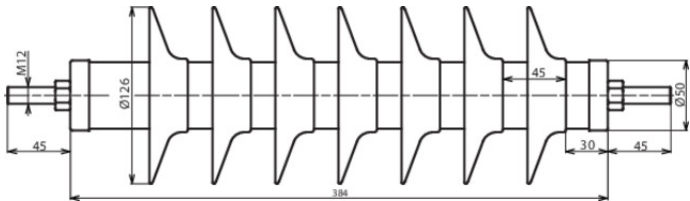
Dimensioni DMI 39 10 1 N
