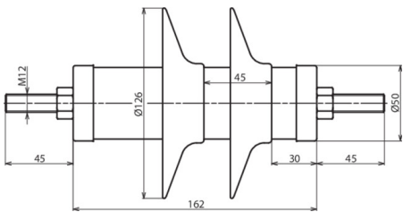
Dimensioni DMI 15 10 1 N
