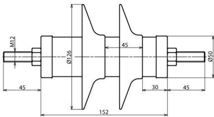
Dimensioni DMI 12 10 1 N
