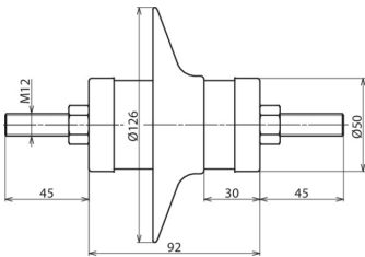
Dimensioni DMI 3 10 1 N
