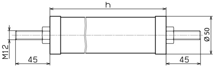
Dimensioni DMI 12 10 1 L
