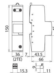
Dimensioni DBM 1 760 FM
