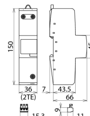
Dimensioni DBM 1 440 FM
