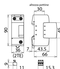
Dimensioni DGP M 255 FM
