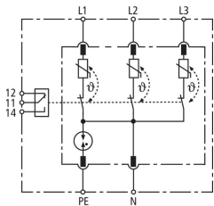
Schema di principio DR M 4P 255 SN1872 FM
