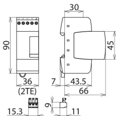
Dimensioni DR M 4P 255 SN1872 FM
