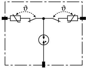
Schema di principio DR MOD 150
