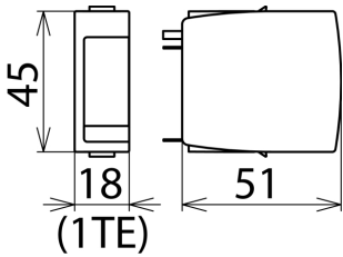
Dimensioni DR MOD 150
