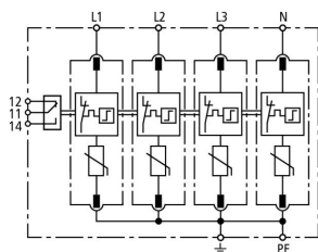
Schema di principio DG M TNS 385 FM
