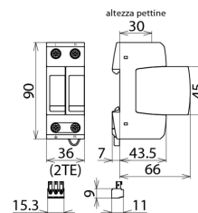
Dimensioni DG M TT 2P 320 FM
