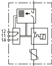
Schema di principio DG S ACI 275 FM
