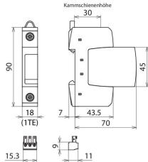
Dimensioni DG S ACI 275 FM
