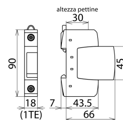
Dimensioni DG S 75 VA
