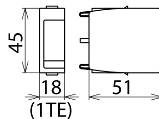
Dimensioni DG MOD PV 600
