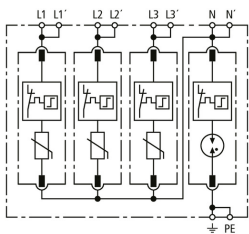
Schema di circuito basilare DG MP TT 275
