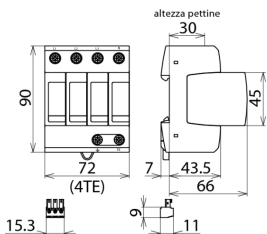
Dimensioni DG MP TT 275
