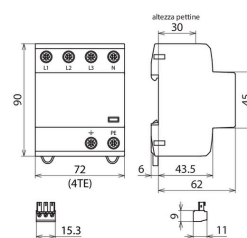
Dimensioni DSH TNS 255 FM
