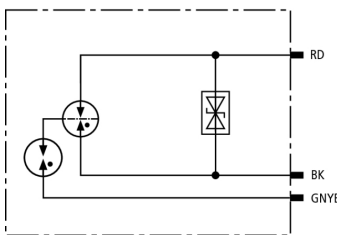
Schema di principio DPI CD EXD 24 M
