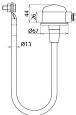
Dimensioni EXFS L100
