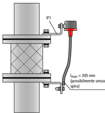
Installazione EXFS L100
