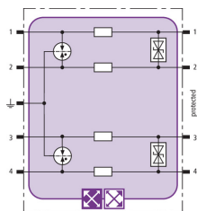
Schema di principio BXT ML4 BD HF 5
