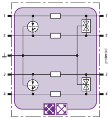
Schema di principio BXT ML4 BE HF 5
