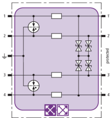
Schema di principio BXT ML4 BC 24
