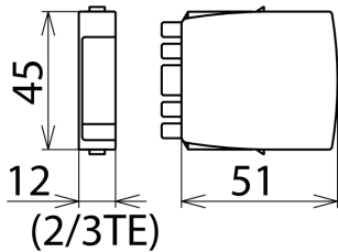
Dimensioni BXT ML4 BC 24
