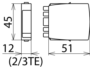
Dimensioni BXT ML4 BD 24
