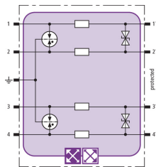
Schema di principio BXT ML4 BD 24
