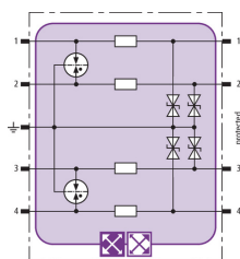
Schema di principio BXT ML4 BE 12
