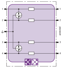
Schema di principio BXT ML4 B
