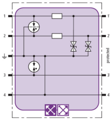
Schema di principio BXT ML2 BE S 12
