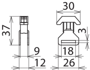
Dimensioni AK 35 SN 18X3 GG
