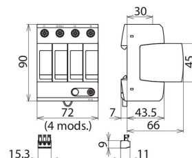
Dimensioni DG MU 3PH 240 4W+G R
