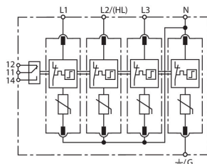
Schema di principio DG MU 3PH 240 4W+G R
