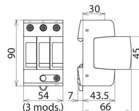
Dimensioni DG MU 3PY 600 3W+G
