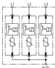
Schema di principio DG MU 3PY 600 3W+G
