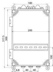
Dimensioni IGA 10 V2 IP54
