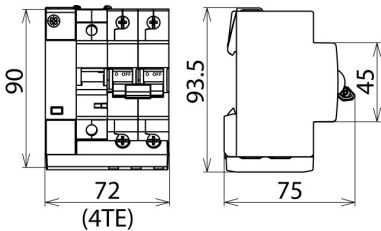
Dimensioni SPD+POP 2 255 C40
