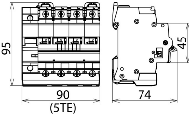
Dimensioni POP 4 255 C25
