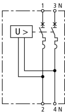
Schema di principio POP 2 255 C40
