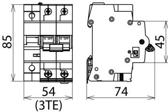
Dimensioni POP 2 255 C40
