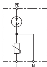
Schema di principio DG TT 2P 5 275
