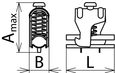
Dimensioni SAK
