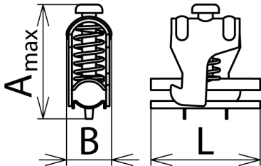
Dimensioni SAK
