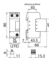
Dimensioni DSE M 1 242 FM
