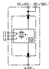
Schema di principio DSE M 1 242 FM
