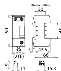
Dimensioni DSE M 1 60 FM
