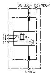
Schema di principio DSE M 1 60 FM
