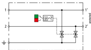
Schema di circuito basilare BCO CL2 E 24
