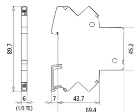
Dimensioni BCO CL2 E 24
